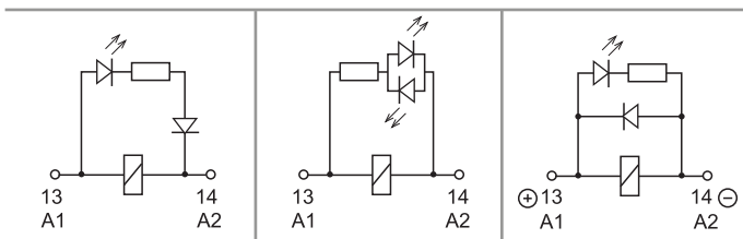
C: Variantes 3, 5, 54 LED (AC) C: Variantes 6, 7, 74 Doble LED (DC no polarizado) C: Variantes 8, 9, 94 LED + diodo (positivo en A1/13, DC polaridad estándar)
